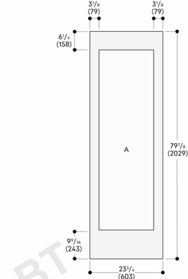
Ширина ниши 24" (610 мм)
